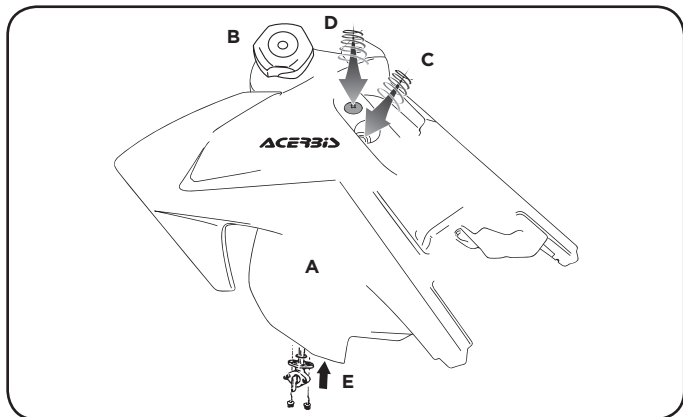
5. Montare il rubinetto (torque spec: 1,8ft/lb 2,5n/m). Posizionare il serbatoio Acerbis. Rimettere la vite-serbatoio. Rimettere la vite sella. Install the petcock (torque spec: 1,8ft/lb 2,5n/m). Place the Acerbis tank. Install the tank screw. Install the seat screw.
