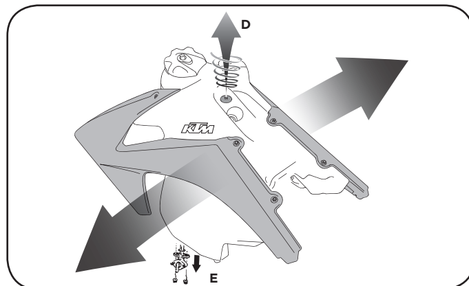
4. Rimuovere la vite-sella. Rimuovere i fianchetti. Rimuovere il rubinetto. Remove the seat screw. Remove the radiator scoops. Remove the petcock
