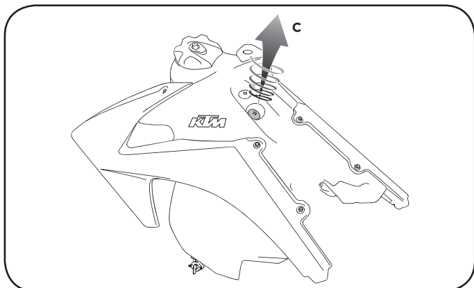
3. Svitare la vite sella. Rimuovere il serbatoio Unscrew the seat screw. Remove the tank
