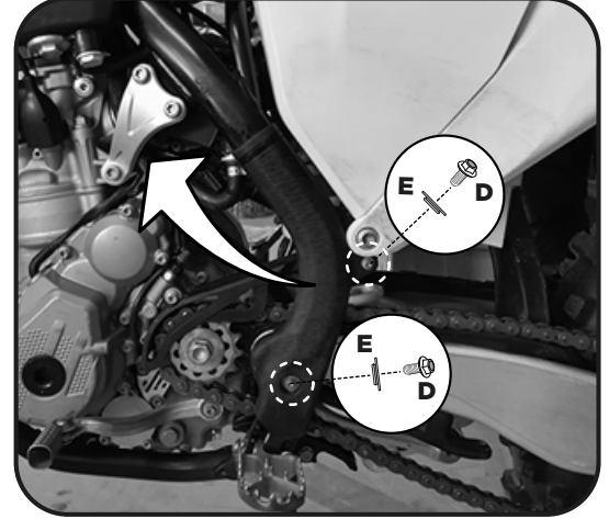
D - (3 pcs.)
